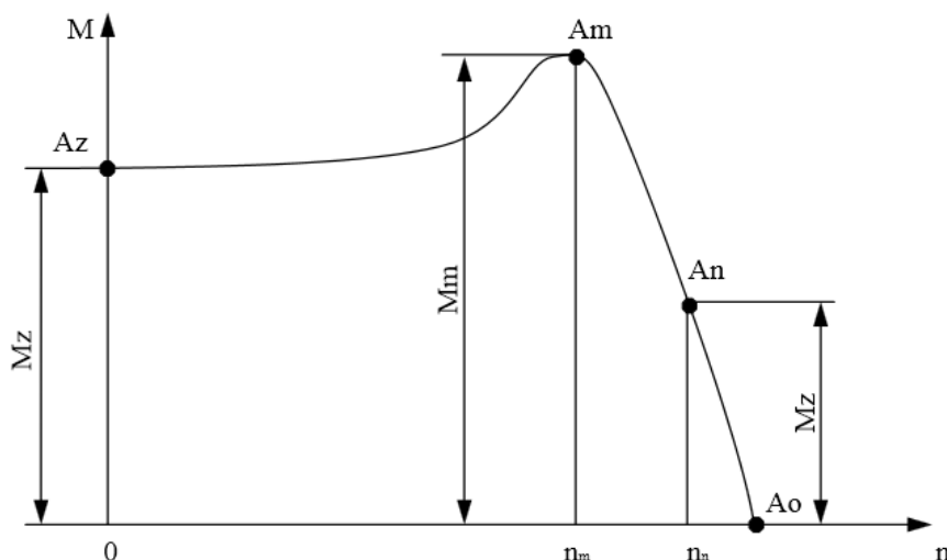
Рисунок 3.1 – Диаграмма зависимости M = f(A.n)
